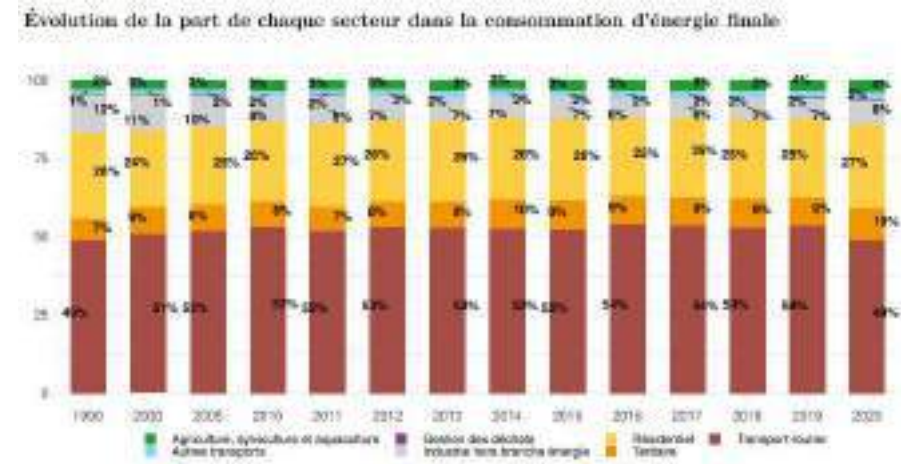
Figure 27 - Evolution de la part de chaque secteur dans la consommation d'énergie finale (ORCAE 2021)
