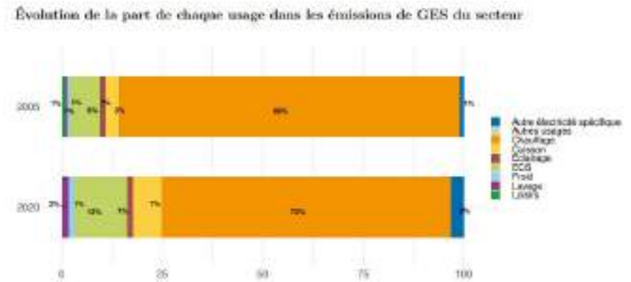
Figure 26 - Evolution de la part de chaque usage dans les émissions de GES du secteur résidentiel (ORCAE 2021)
