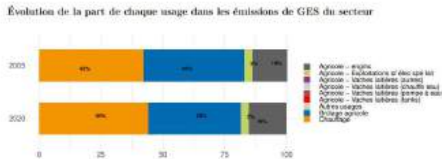
Figure 25 - Evolution de la part de chaque usage dans les émissions de GES du secteur agricole (ORCAE 2021)
