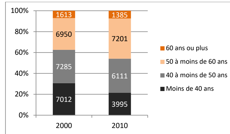
Figure 15 – SAU en fonction de l'âge du chef d'exploitation en 2000 et 2010
