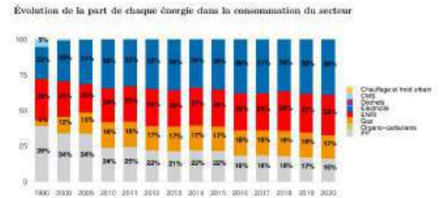
Figure 30 - Evolution de la part de chaque énergie dans le secteur résidentiel (ORCAE 2021)
